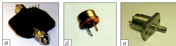
Рис. 3. Мініатюрні прецизійні перетворювачі тиску: a — для обліку витрат природного газу; б — для дистанційного контролю тиску в автомобільних шинах; в — для газодинамічних випробувань ракетно-космічної техніки
